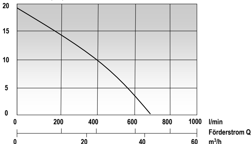
Förderhöhe H m (WS)
